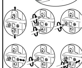
Установка и регулировка петель
