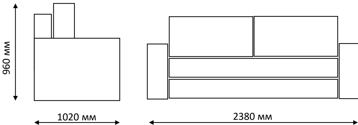
Габаритные размеры
